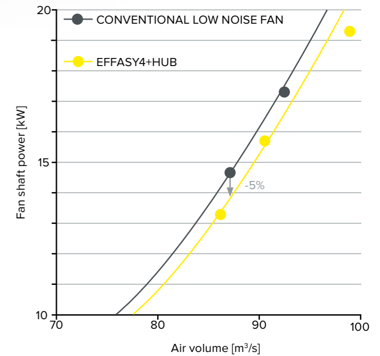
EFFASY fan - Fan shaft power
